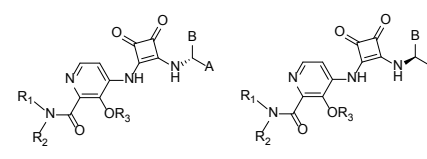
Fórmula (IA)
